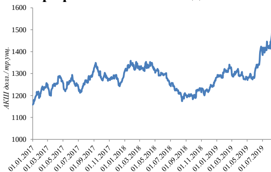
1.2.4-график. Алтынга баа динамикасы
