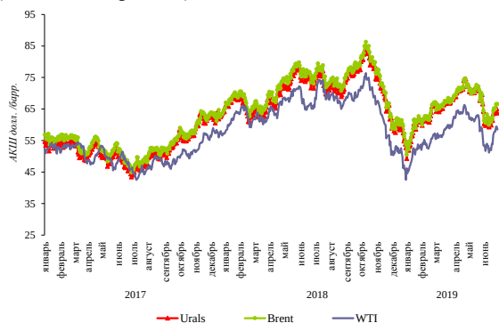
1.2.3-график. Мунайга баанын динамикасы (АКШ долларында)
