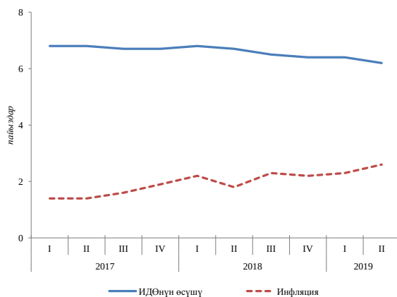
1.1.6-график. Кытайда ИДӨнүн жана инфляциянын өсүш динамикасы (өткөн жылдын тиешелүү чейрегине карата чейрек)
